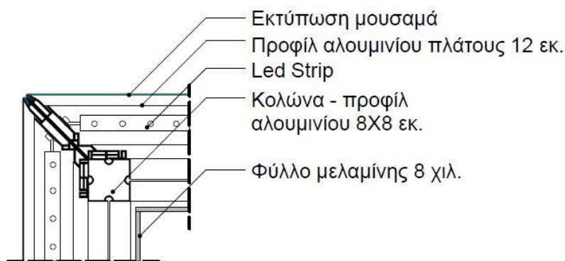
ΛΕΠΤΟΜΕΡΕΙΑ ΚΑΤΑΣΚΕΥΗΣ
