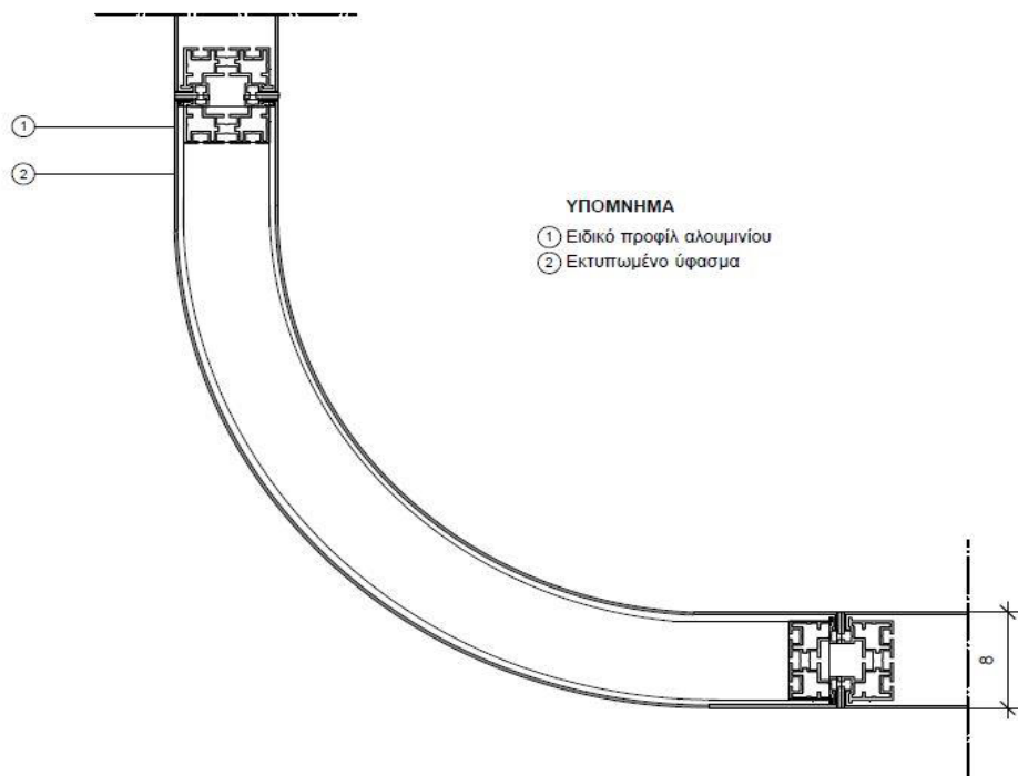
ΚΑΤΟΨΗ, ΚΛΙΜΑΚΑ 1.5 ΚΑΤΑΣΚΕΥΑΣΤΙΚΗ ΛΕΠΤΟΜΕΡΕΙΑ ΑΝΑΡΤΗΜΕΝΗΣ ΚΑΤΑΣΚΕΥΗΣ ΟΡΟΦΗΣ
