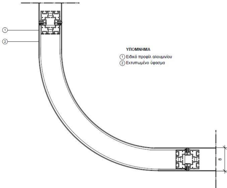
ΚΑΤΟΨΗ, ΚΛΙΜΑΚΑ 1.5 ΚΑΤΑΣΚΕΥΑΣΤΙΚΗ ΛΕΠΤΟΜΕΡΕΙΑ ΑΝΑΡΤΗΜΕΝΗΣ ΚΑΤΑΣΚΕΥΗΣ ΟΡΟΦΗΣ
