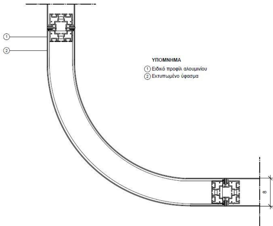
ΚΑΤΟΨΗ, ΚΛΙΜΑΚΑ 1.5
