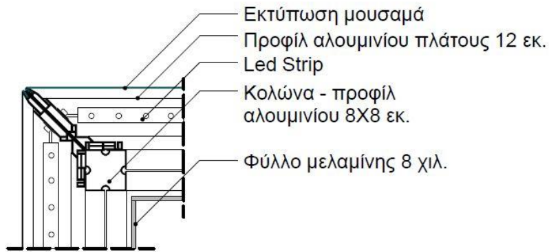
ΛΕΠΤΟΜΕΡΕΙΑ ΚΑΤΑΣΚΕΥΗΣ
