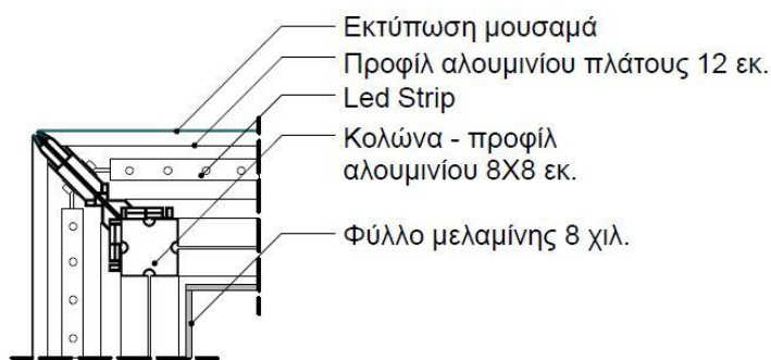
ΛΕΠΤΟΜΕΡΕΙΑ ΚΑΤΑΣΚΕΥΗΣ
