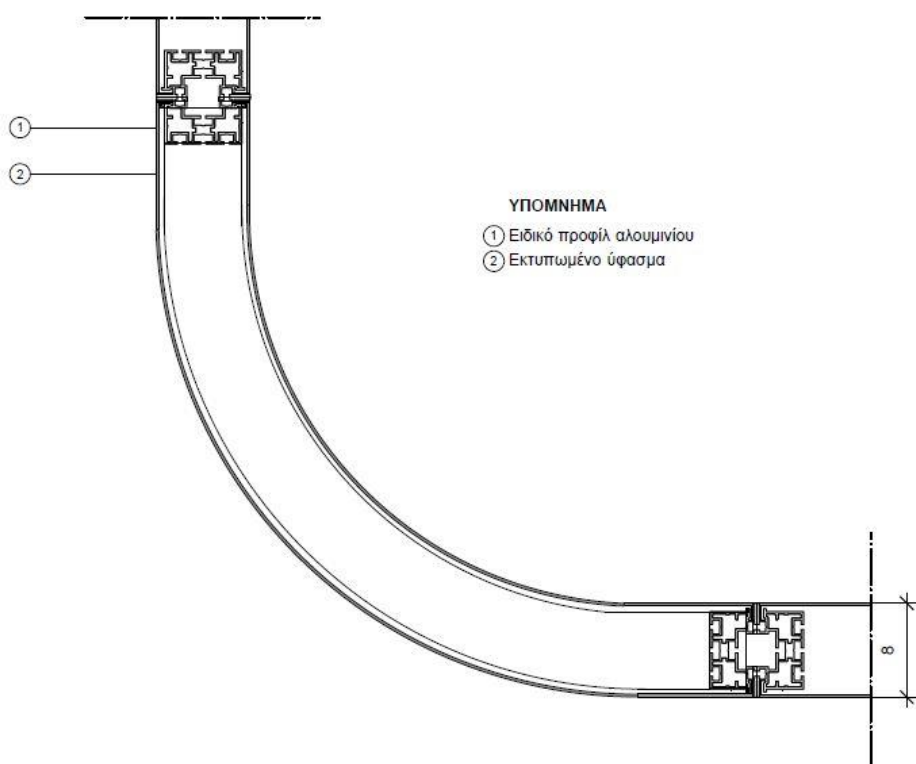
ΚΑΤΟΨΗ, ΚΛΙΜΑΚΑ 1.5
