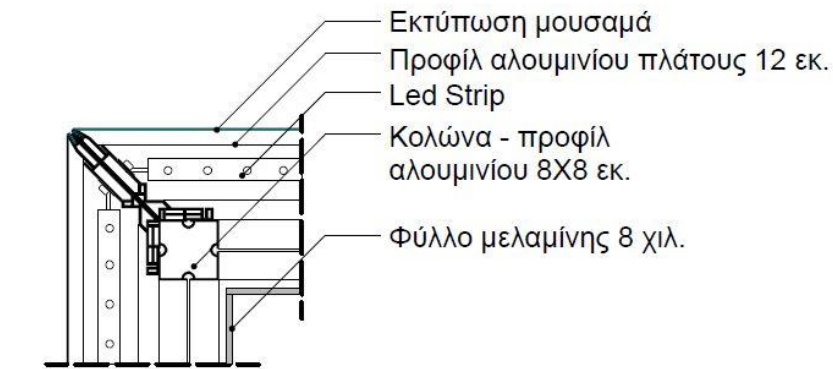
ΛΕΠΤΟΜΕΡΕΙΑ ΚΑΤΑΣΚΕΥΗΣ
