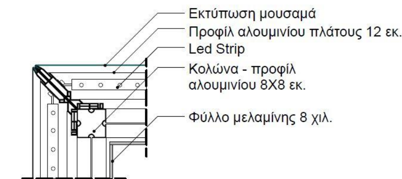
ΛΕΠΤΟΜΕΡΕΙΑ ΚΑΤΑΣΚΕΥΗΣ
