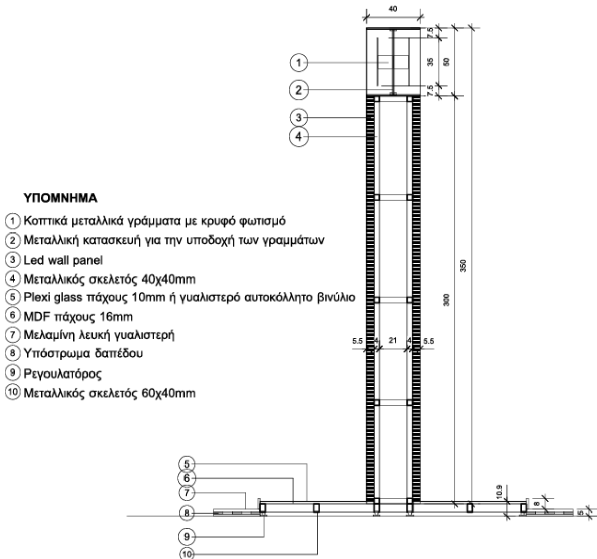
ΚΑΤΑΣΚΕΥΑΣΤΙΚΗ ΛΕΠΤΟΜΕΡΕΙΑ LED WALL
