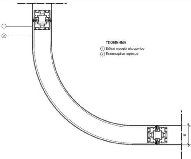
ΚΑΤΟΨΗ, ΚΛΙΜΑΚΑ 1.5
